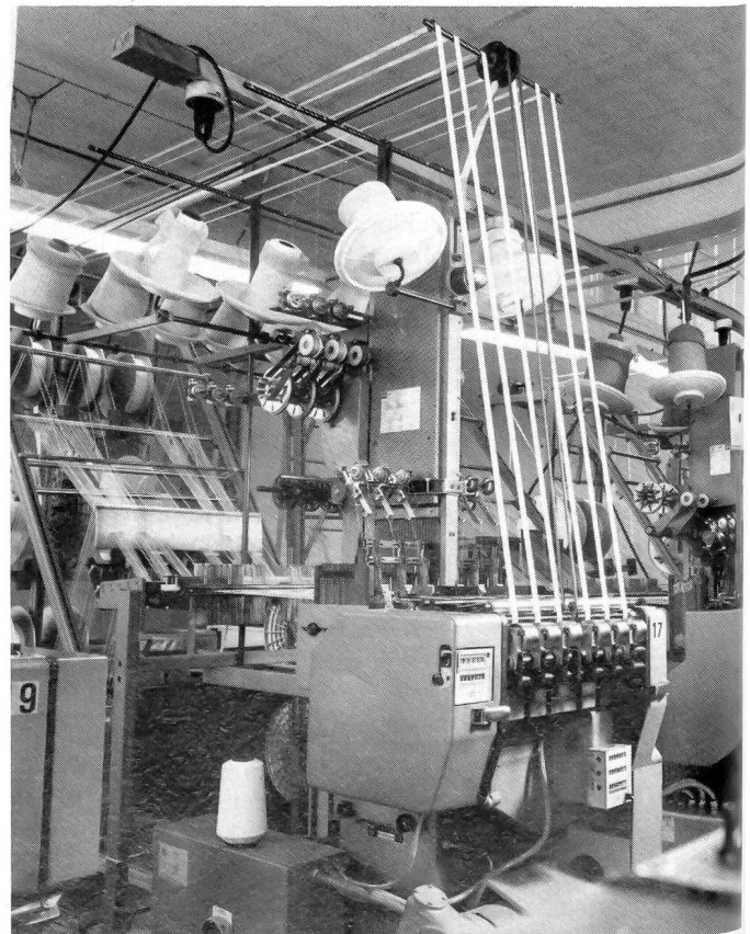
Teilansicht eines modernen Webautomaten für Schaffbänder mit einer Leistung von über 2000 Trs./Min.
