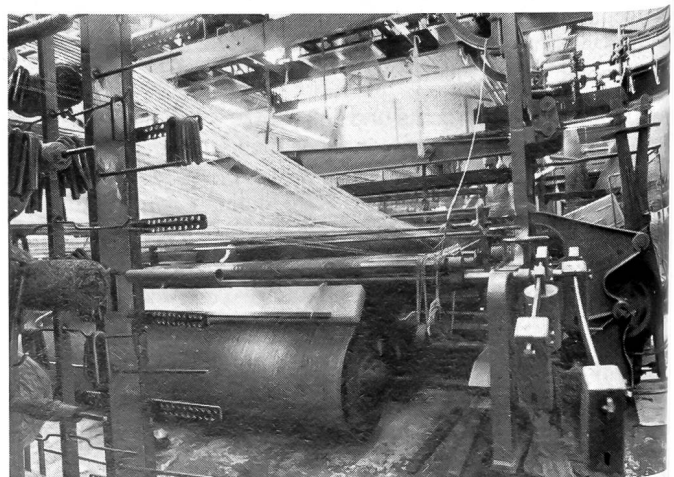
3 Ansicht einer Rutenwebmaschine
