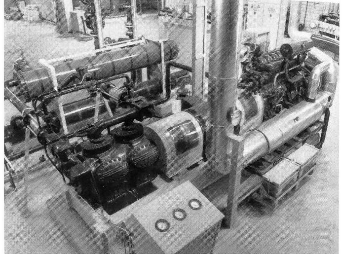
6. Tandem-Anlage bei Siemens, Heidenheim. Links hinten Verdampfer und Kondensator, vorne der Wärmepumpenkompressor, hinter dem Abgas-Sammler der Elektromotor/Generator, rechts der Gasmotor.
