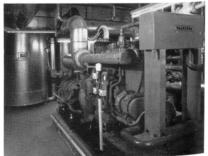
8. Gas-Wärmepumpe zur Wärme- und Kälteerzeugung im WfG-Gebäude in Dortmund.
