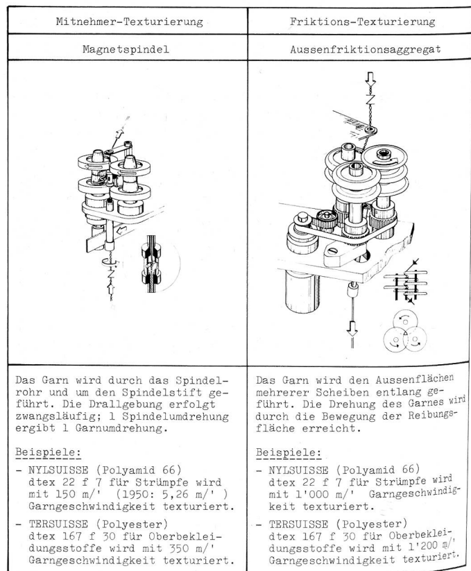
Abbildung 2 Mittnehmer- und Frikions-Texturierung
