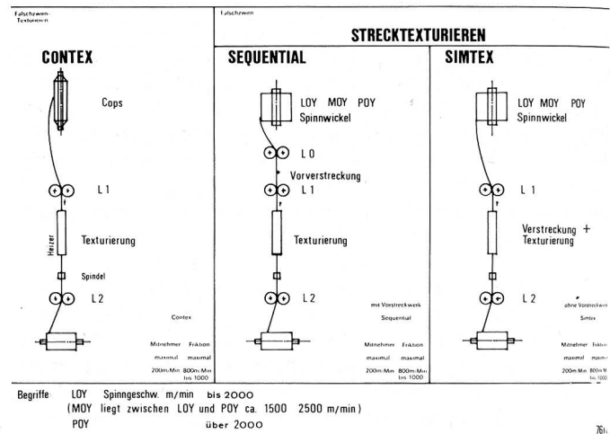
Abbildung 2 Mittnehmer- und Frikions-Texturierung
