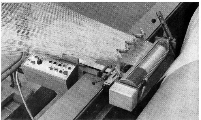
Abb. 6 Regelduo
