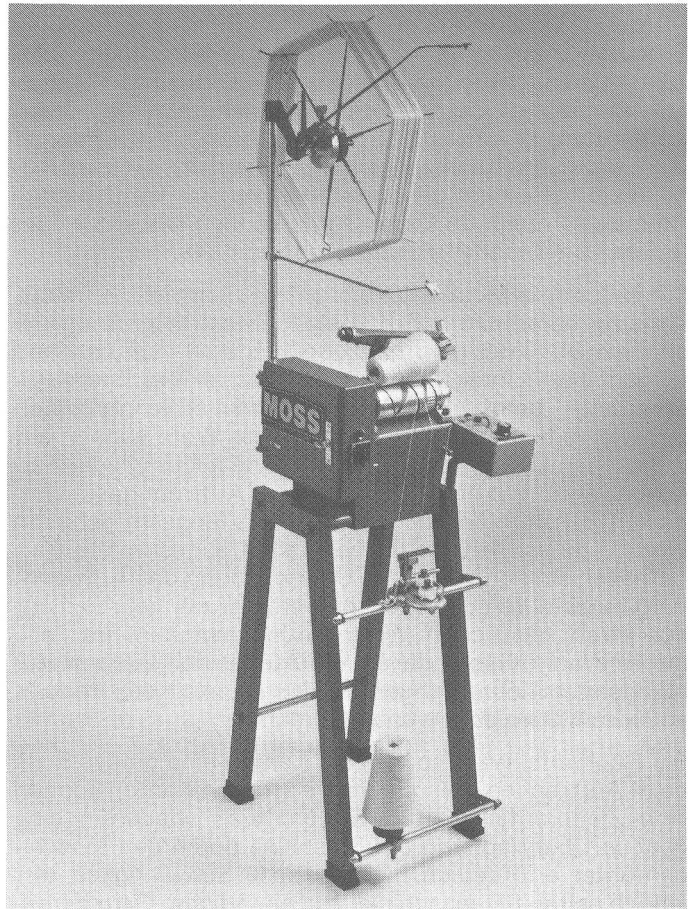
Die freistehende Ausführung der auch als integrierter Bestandteil der Grundausführung des «Backwinder» erhältlichen Strang-Kegel-Aufspulmaschine von Moss.
