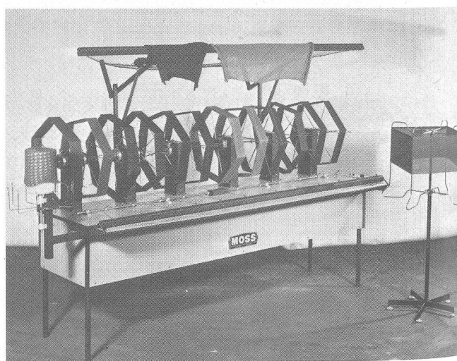
Die mit 12 Systemen ausgerüstete Strickwaren-Auftrennmaschine des von der Firma Moss hergestellten «Backwinder». Das spezielle Auftrennkarussell für Rundstrickware steht rechts daneben.
