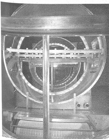
Serienmontage von vor- fabrizierten Sulzer Hochleistungs-Luftwäschern mit automatischem Wasser- filter für Textilklimaanlagen.
