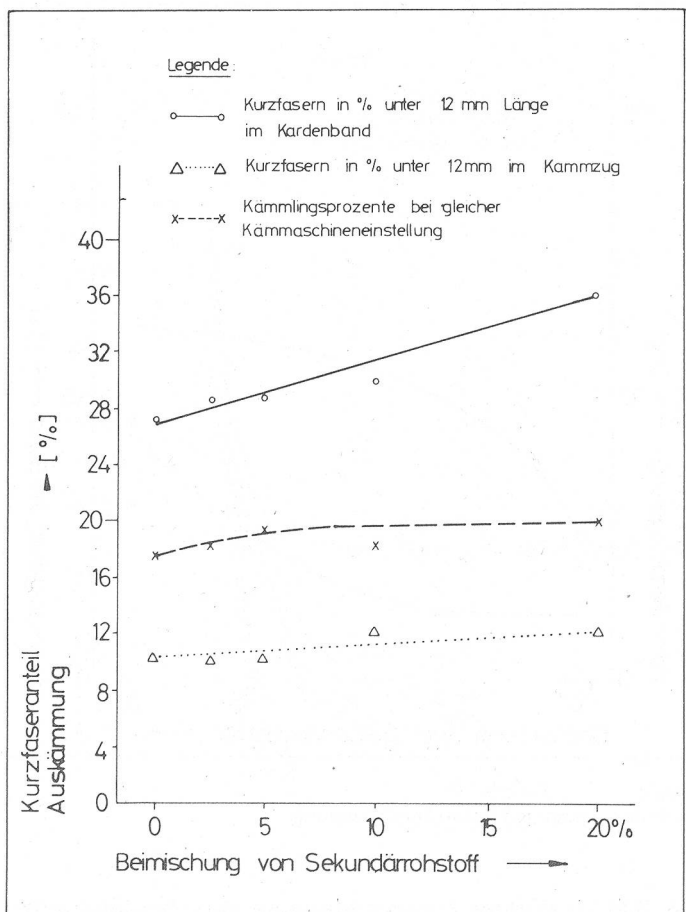
Bild 3: Auskämmung und Kurzfaserteil
