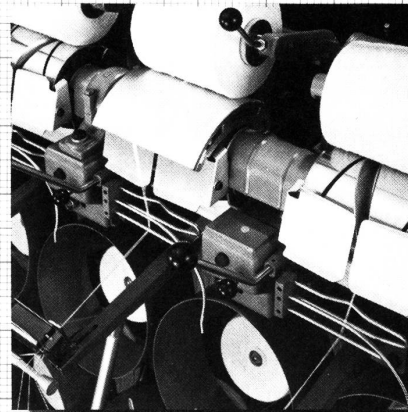
FMX mit wilder Wicklung und piezo-elektronischer oder elektro-mechanischer Fadenüberwachung
