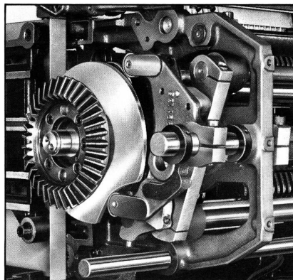
Komplementär-Kurvenscheiben auch für den Antrieb der Abstümmesser 3 mit neuartiger Doppelfunktion: für die zwangsläufige Steuerung der Zughaken 2 und für die spielfreie Verriegelung der nicht arbeitenden Zughaken.
