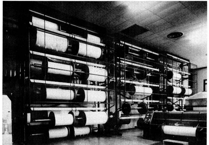
Bild 1: Drei Vertikalständer, Kettbaumdurchmesser 800 mm, Kettbaumbreite 1850 mm, Kettenabstand 4200 mm, Kettbaumgewicht 400 kg, Gesamtgewicht 9600 kg, Fassungsvermögen je 12 Tragegängen = 24 Kettbäume. Masse eines Ständers: Breite 4520 mm, Tiefe 1886 mm, Höhe 7570 mm, Ständer mit Schutzgitter versehen.
