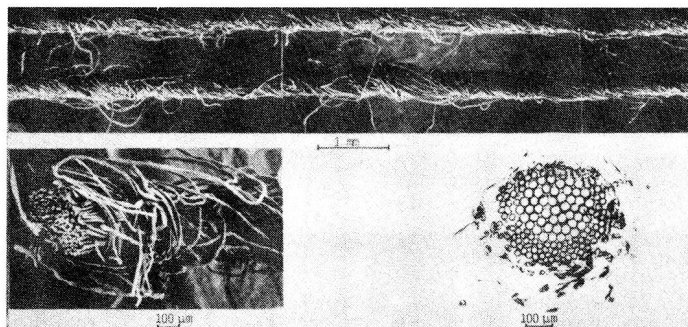
Abb. 3 REM-Aufnahmen und lichtmikroskopische Querschnittaufnahme eines OE-Friktionsspinnagarns (DREF) 55 tex, Filament (180 dtex)/Baumwolle
