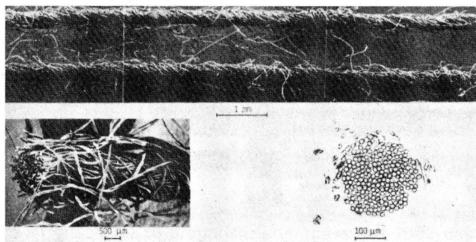
Abb. 2 REM-Aufnahmen und lichtmikroskopische Querschnittaufnahmen eines OE-Friktionsspinnagarns (DREF) 50 tex, 60% Kern (PES)/40% Mantel (Baumwolle)
