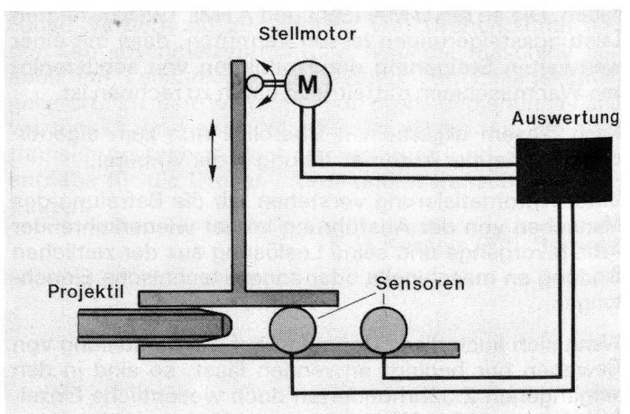
Projektilebremse (selbstregulierend)
