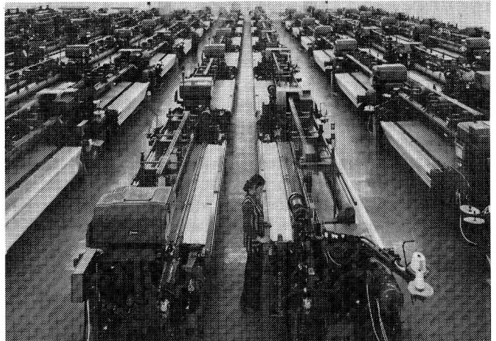
Der 1971 neu erstellte Websaal ist mit 98 Rütli C-Schützenmaschinen, alle mit Unifil und elektronischen Schützenflugmaschinen dotiert. Eine Weberin hat hier 24 der breiten Maschinen zu bedienen.
