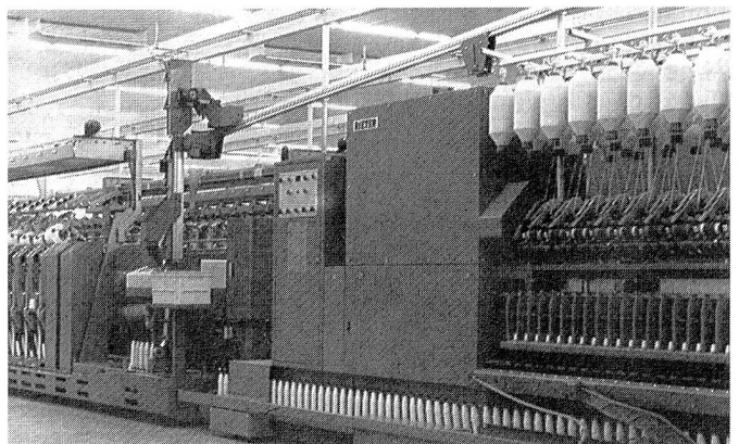
Ringspinn-Spulmaschine
