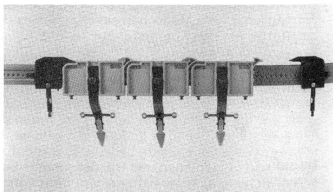
Die Abbildung zeigt den Anwendungsfall als Mehrfachkasten; drei Fadenführerkästen arbeiten auf einer Spür zusammen.
