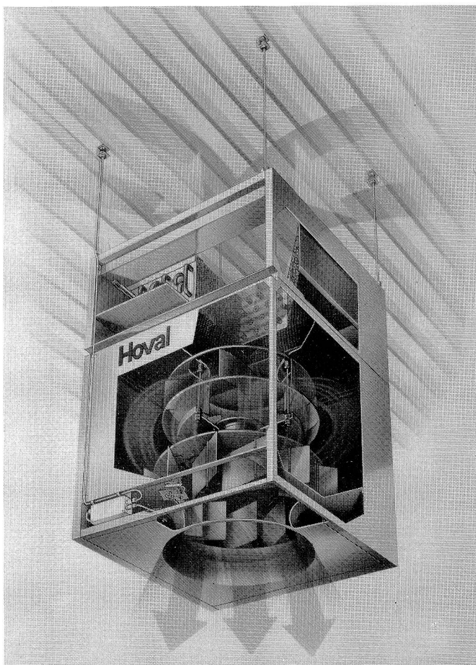
Hoval DHV-Gerät: Decken-Umlufttheizgerät für Industrie und Gewerbe (Werkphoto Hoval)
