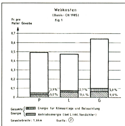
Anteil der Energiekosten an den Webkosten Quelle: Sulzer Rütli
