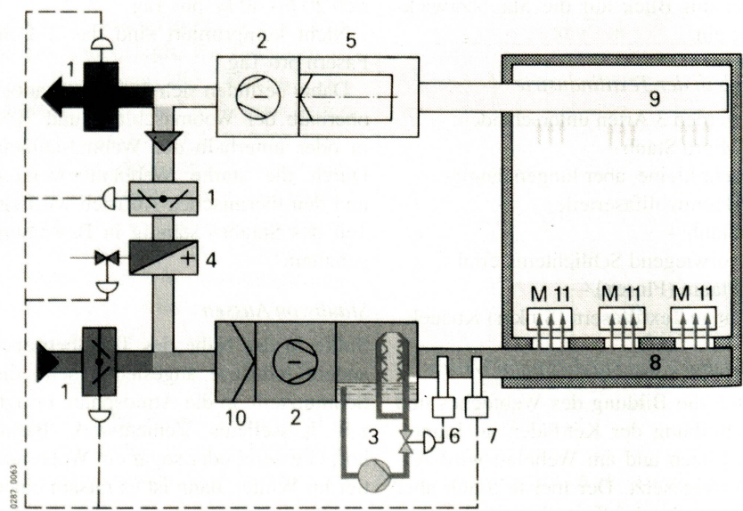
Condifil Klimasystem, M = Textilmaschine, 1 = Regelklappe, 2 = Ventilator, 3 = Luftwäscher, 4 = Lufterhitzer, 5 = Abluftfilter, 6 = Feuchtefühler, 7 = Temperaturfühler, 8 = Zuluft, 9 = Abluft Grafik: Sulzer Infra
