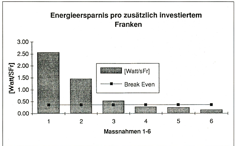
Wirtschaftlichkeit von Energiesparmassnahmen. 1 = Klimafilter, 2 = Wetter-schutz, 3 = FDA-Filter, 4 = Zuluft-Kanalsystem, 5 = Frequenzumformer Wascherpumpe, 6 = Waschervolumen
