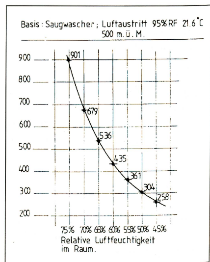
Die Grafik zeigt das Kühlvermögen gesättigter Luft resp. den Kühlluftbedarf in m³/h pro kW freigesetzter Wärme bei entsprechender relativer Luftfeuchtigkeit im Raum.
