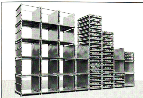
Flexible Produktions-Lager mit beladenen und leeren DRAWAG-Schwerlastpaletten
