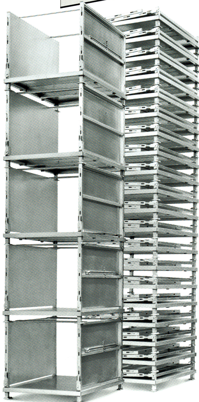
Sicheres Stapeln von 5 beladenen oder 20 leeren DRAWAG-Schwerlastpaletten
