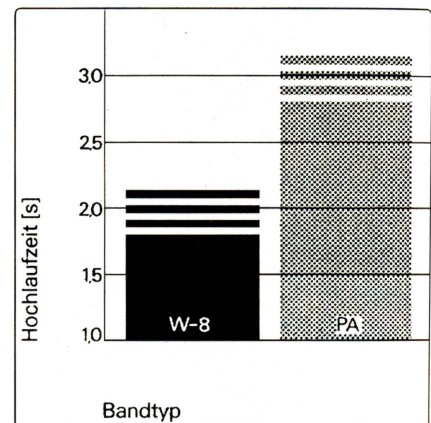
Abb. 2: Minimierte Hochlaufzeit durch verbessertes Adhäsionsverhalten
