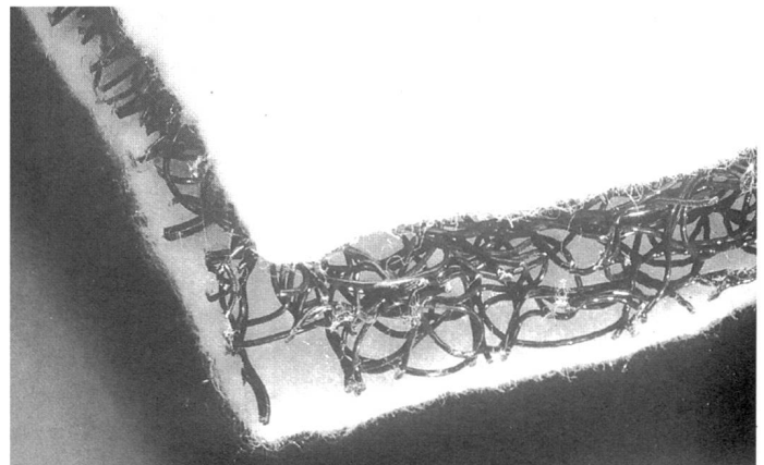
Abb. 2: Vlies-3D-Strukturmatte
