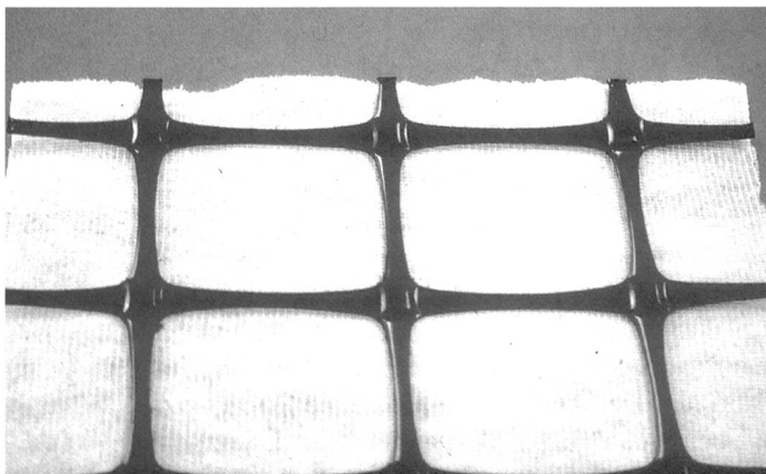
Abb. 1: Vlies-Geogitter-Kombinationen
