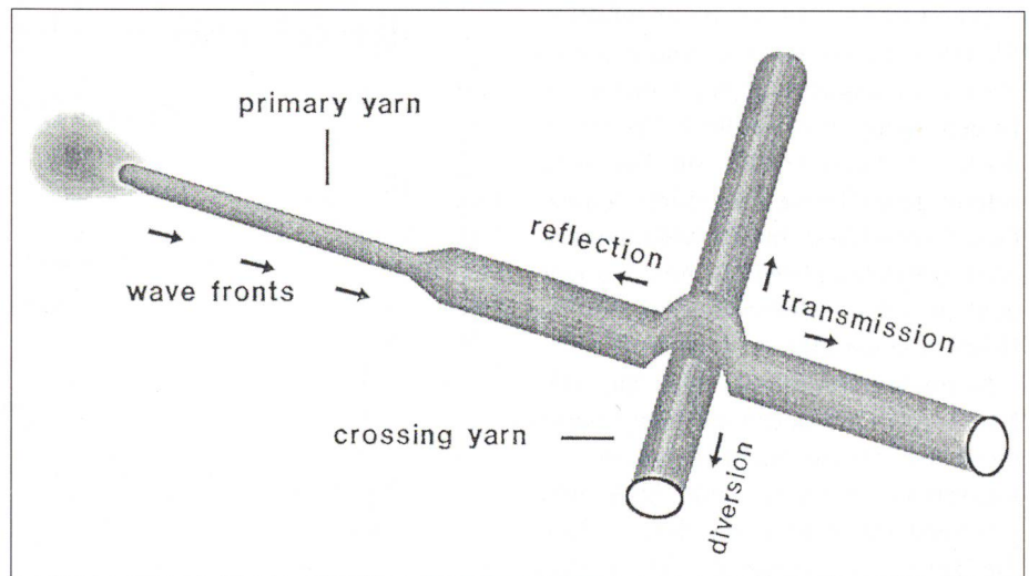
Abb. 1: Schockwellenfortpflanzung im Gewebe nach einer ballistischen Einwirkung
