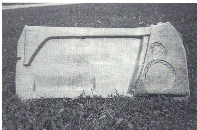
Bild 6: Türinnenverkleidung
