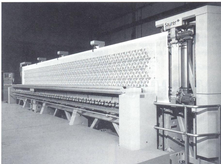
Stickmaschine Saurer EPOCA
