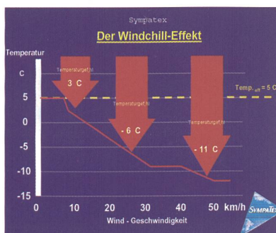
Abb.: 1 Windchill-Effekt
