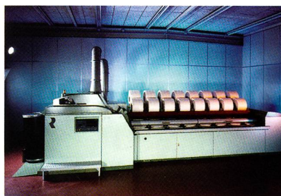
Abb. 2: Kämmaschine E 72
