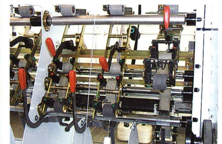
Fashionator – Streckwerk
