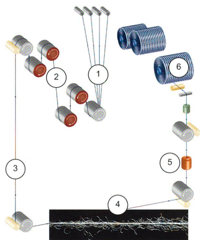
Der Uniplex™-Prozess
