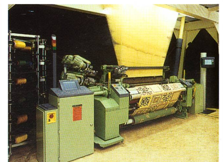
Luftdüsenwebmaschine AWSL 4 mit selbstangetriebener, oberbauloser Drehereinrichtung EasyLeno ®
