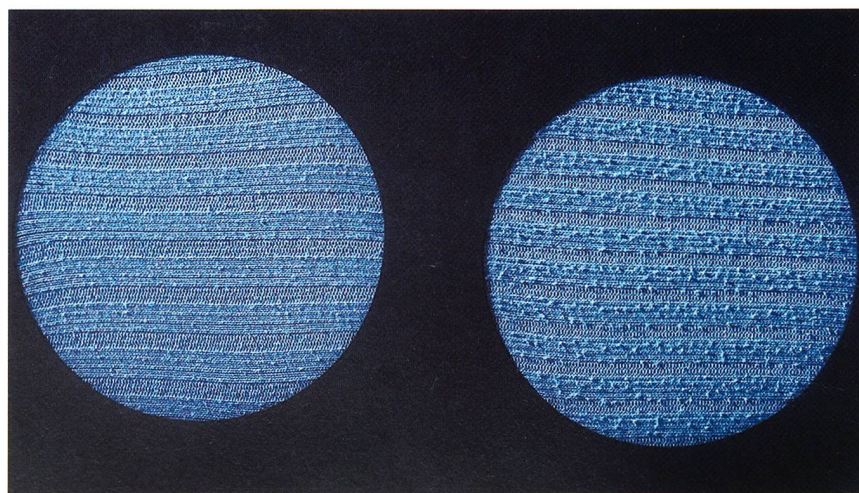
Rundgestrick in Rippsbindung aus 100 % pillbeständigem Polyester nach 5'000 Scheuerzyklen, links mit Futura®-Garnen, rechts mit konventionellen Ringgarnen
