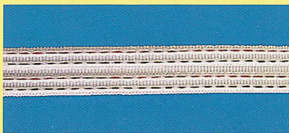
Textiles Band für die Datenübermittlung in Smart-Textiles mit im Schmalgewebe eingebetteten Multifilamenten aus Metalldraht, hergestellt von der Elekrisola Feindraht AG (Escholzmatz, Schweiz), Bildnachweis: Elekrisola Feindraht AG
