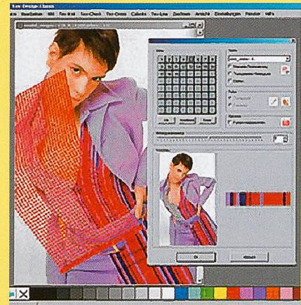
Tex-Dress / Koppermann
