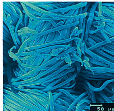
Abb. 2: Kritische Faserenden können Hautunverträglichkeitsreaktionen auslösen
