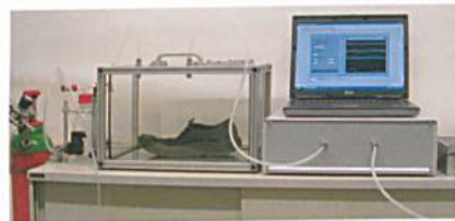
Abb. 2: Mit Hilfe der so genannten «Elektronischen Nase» soll künftig bereits bei der Entwicklung von Schuhen und Strümpfen das Potential für unangenehmen Schweißgeruch abschätzbar sein, Bild: PFI Pirmasens
