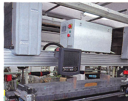
Abb. 3: UNIVALETTE für das Namenseinweben in Webleisten
