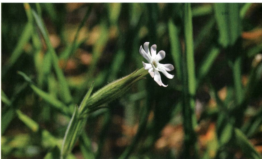
Abbildung 1: Unter den gefährdeten Arten sind auffällig viele Ackerwildkräuter zu finden. Arten wie die Acker-Lichtnelke (Silene noctiflora L.) kamen in mehreren Untersuchungsflächen vor. Foto: Thomas Stalling.
