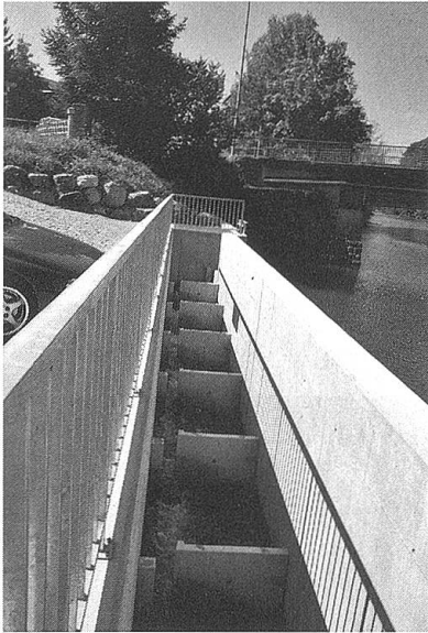
Fischtreppe in der Mühlau.
