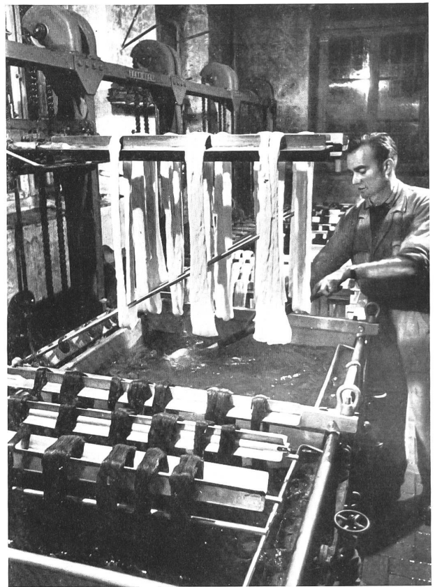
Strangfärbemaschine für Seidenzwirne. Zwicky & Co., Wallisellen.
