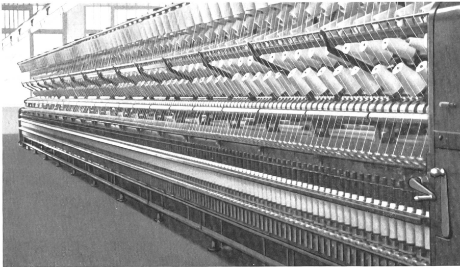
Generalansicht einer Baumwoll-Ringzwirnmachine. Bäumlin, Ernst & Co., St-Gallen.
