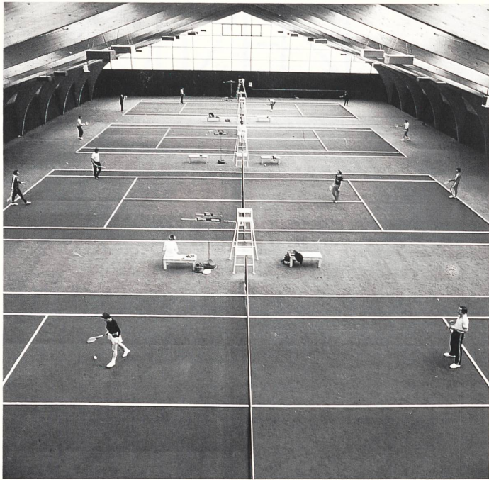
Erster Schweizer Tennis-Velours – ein speziell für Sporthallen entwickelter Tennisboden aus 100% Swiss Polyamid-Grilon® im Sportzentrum Pfäffikersee in Pfäffikon/ZH.
