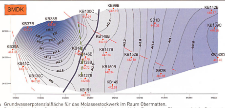
Fig. 10: Grundwasserpotenziellfläche für das Molassestockwerk im Raum Obermatten. Dunkelblaue Linie: Grundwasserscheide, gestrichelte rote Linie: Begrenzung Rinnensandstein Ost, gestrichelte grüne Linie: Interventionsbrunnenreihe in der darüberliegenden Kölliker Rinne. Massstab: CH-Koordinatennetz.
