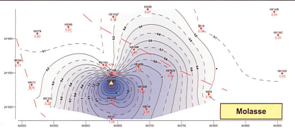
Fig. 13: Absenktichter in der Molasse (Rinnensandstein Ost) und im Lockergestein der Kölliker Rinne nach 300h Pumpbetrieb in KB1288 (Brunnen im Rinnensandstein mit Q=12 \text{ l}/\text{min} ). Die Darstellung erfolgt mittels Isolinen und Messwerten, welche die Potenzialreduktion in [m] darstellen. Massstab: CH-Koordinatennetz.
