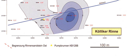
Fig. 12: (links); Reduktion der el. Leitfähigkeit in \mu\text{S}/\text{cm} nach 30-tägigem Pumpbetrieb in KB1288. Blaue Zonen: markanter Rückgang der el. Leitfähigkeit. Rote Strichlinie: Begrenzung Rinnensandstein Ost. Massstab: CH-Koordinatennetz.
