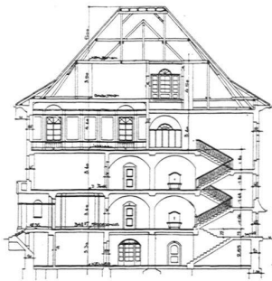
Querschnitt Primarschule 1 : 600
