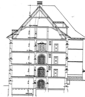
Querschnitt Sekundarschule 1 : 600
