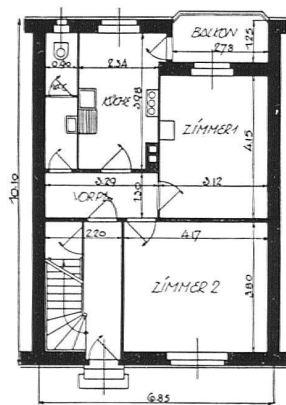
ERDGESCHOSS REZ-DE-CHAUSSÉE
