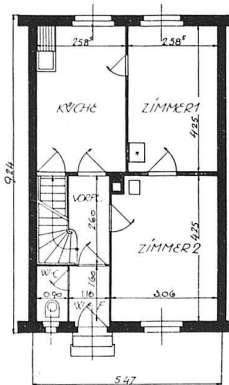
ERDGEHOIS RÉZ-DE-CHAUSSÉE
