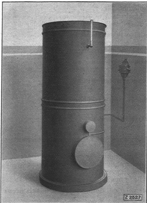
Elektrischer Warmwasser-Apparat mit Heizwiderständen. Gebaut in Grössen von 100 bis 1000 Liter Inhalt und 1,5 bis 11 KW Anschlusswert.
