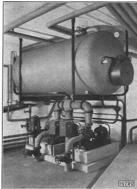
Elektrische Warmwasserbereitungsanlage in einem grossen Spital. Speicher von 3000 Liter Inhalt, Anschlusswert 30 KW.
