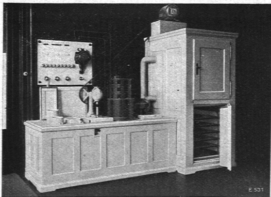
Abb. 5. Kühleinrichtung mit Autofrigor A 1203 für Hotels und Konditoreien zur Eiszerzeugung und gleichzeitigen Raumkühlung.
