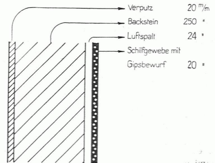
Abb. 9. Backsteinmauer, aussen verputzt, innen mit Schilfwergewebelag und Gipsbewurf.
