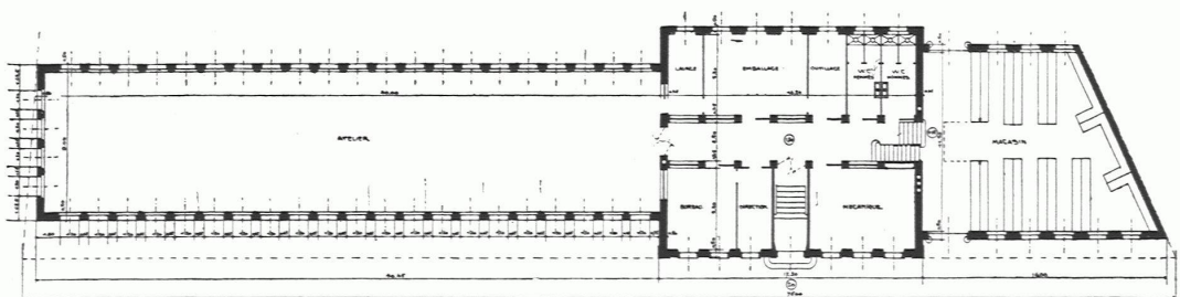
PLAN DU REZ-DE-CHAUSSEE
