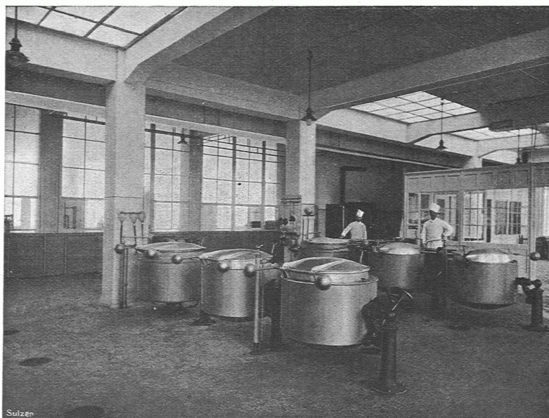
Dampfküche mit 18 Sulzer-Kochkesseln von zusammen 2100 Liter Inhalt, für 0,4 Atm. Betriebsdruck.
