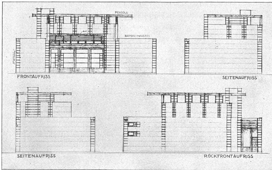
Aufnisse des Einheitshauses
