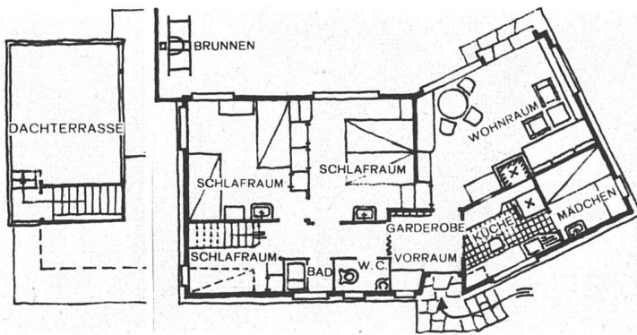
Obergeschoss Erdgeschoss 1:200
