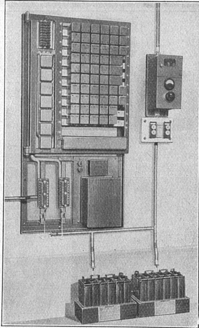
Automatische Hauszentrale „Hasler“ für 25 Teilnehmer
